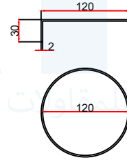
POLE CAP
