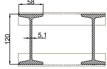
SECTION A-A SCALE : 1/5
