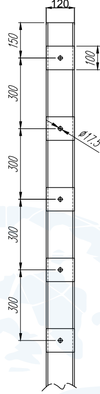
SECTION B-B SCALE : 1/15
